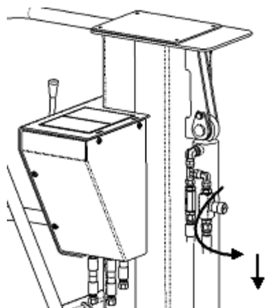
Valvola di discesa di emergenza sulla piattaforma
